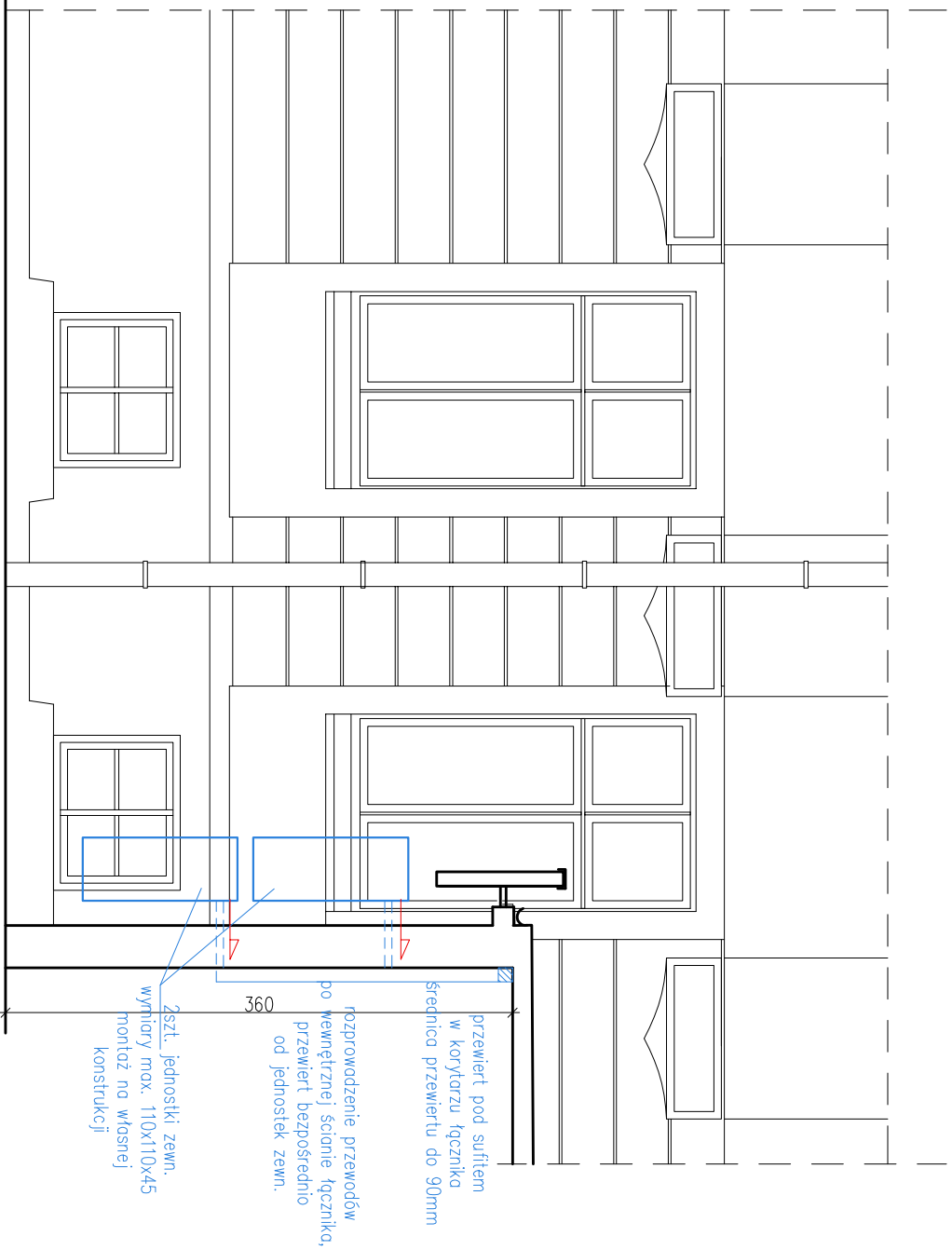
WIDOK 6-6
